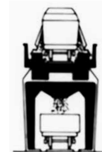
Entladebrücke # 61122 Unloading gantry # 61122 / Ponte de déchargement # 61122 / 卸货装置 # 61122
